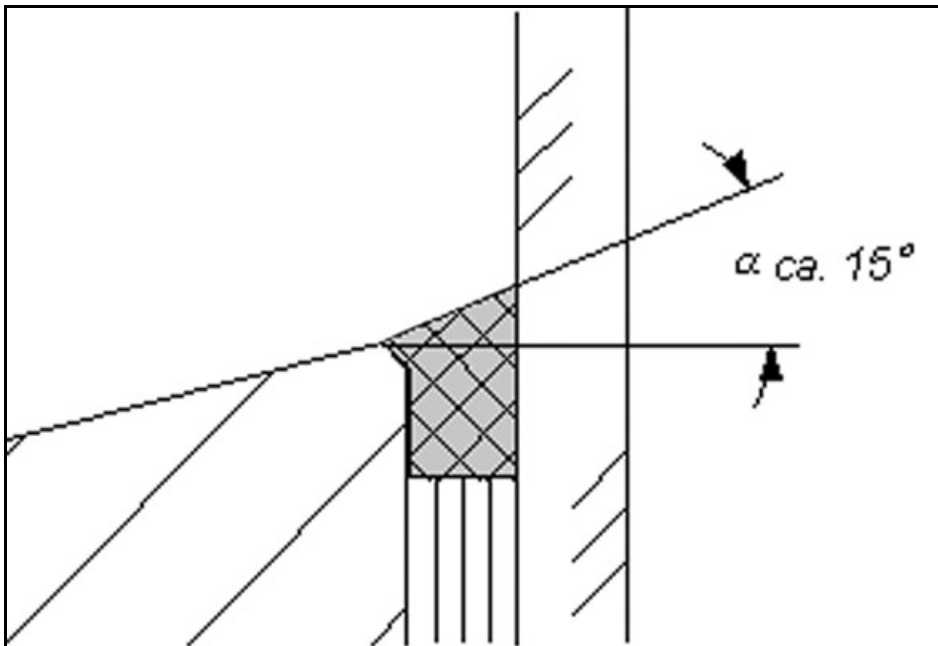
Beispiel: Dichtstoffgeometrie der Versiegelung Verglasung mit Vorlegeband
