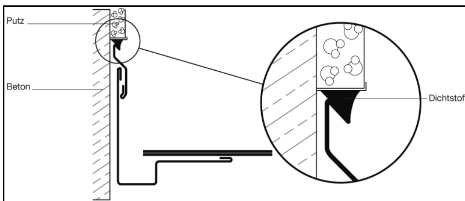
Beispiel: Anschluss Überhangstreifen
