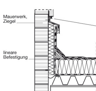
Bauteilfugen und Fugen an Fenster und Fassade
